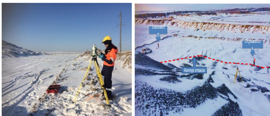
13 Сурет – T1 станциясында тахеометрмен жұмыс
