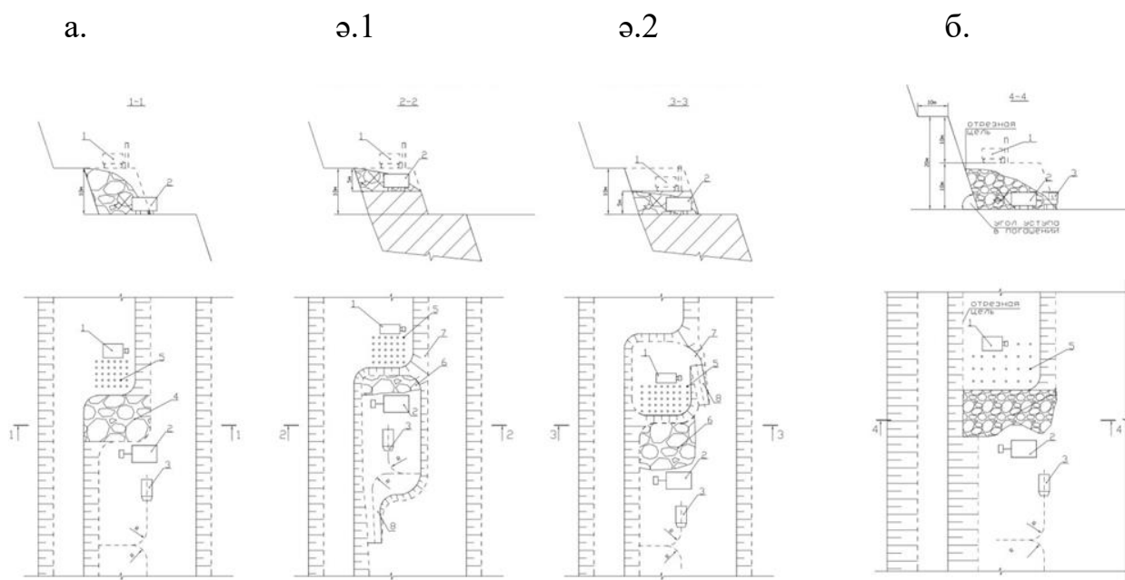
2 Сурет – Кемерде жұмыс істеудің технологиялық сұлбалары
