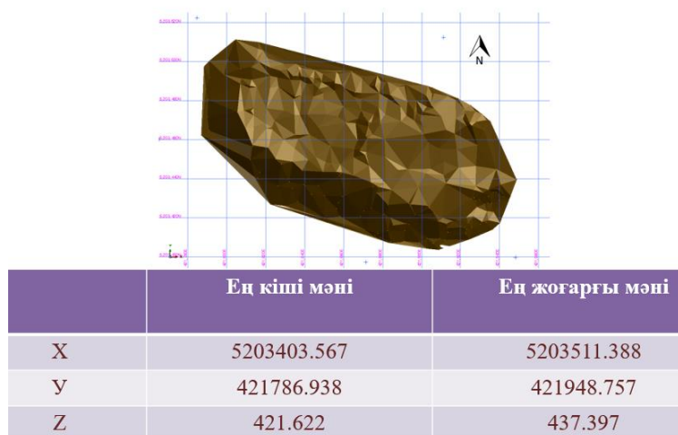
14 Сурет – Сандық топографиялық модель
